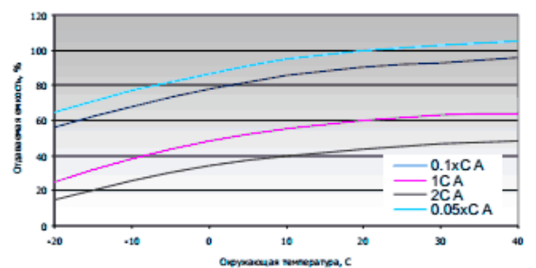
Зависимость емкости от температуры
