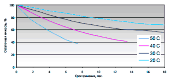
Характеристики саморазряда
