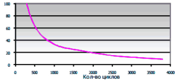
Зависимость кол-ва циклов от глубины разряда (GEL)
