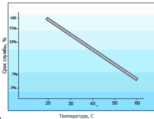
Зависимость срока службы от окружающей температуры
