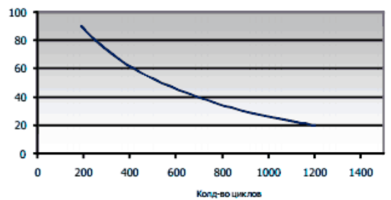
Зависимость кол-ва циклов от глубины разряда (AGM)
